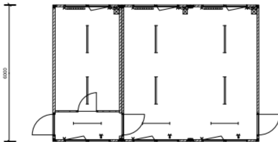
Verdieping
